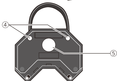
フロアレーザー本体底面
